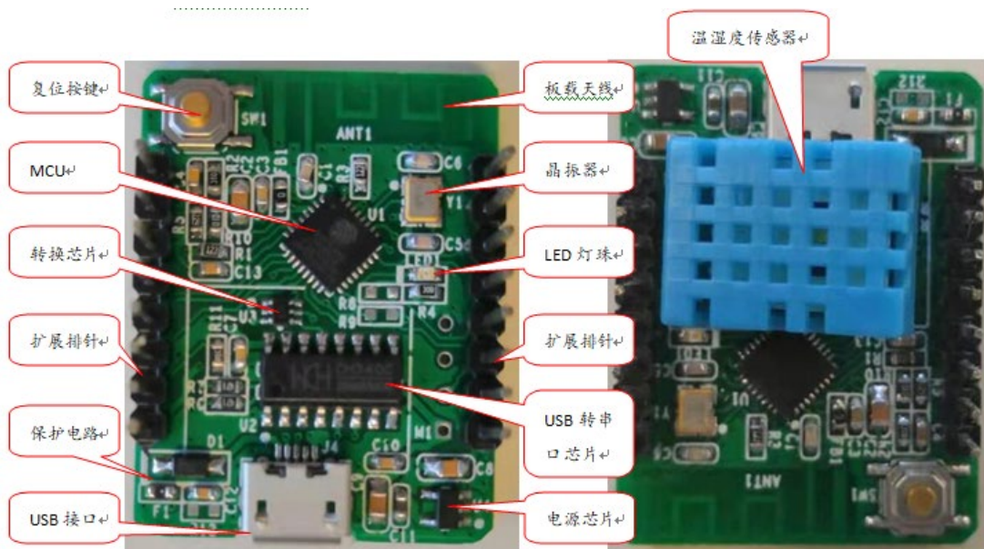
图 14 微型开发板资源图
